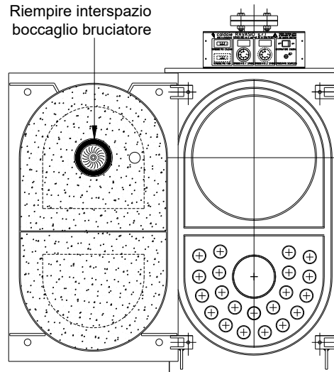
Vista frontale caldaia con portellone aperto.
